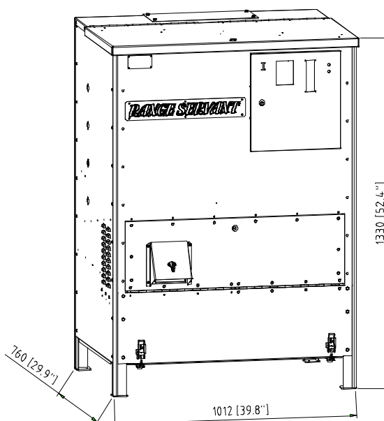
Figur 2: Bollautomat Ultima-8.
