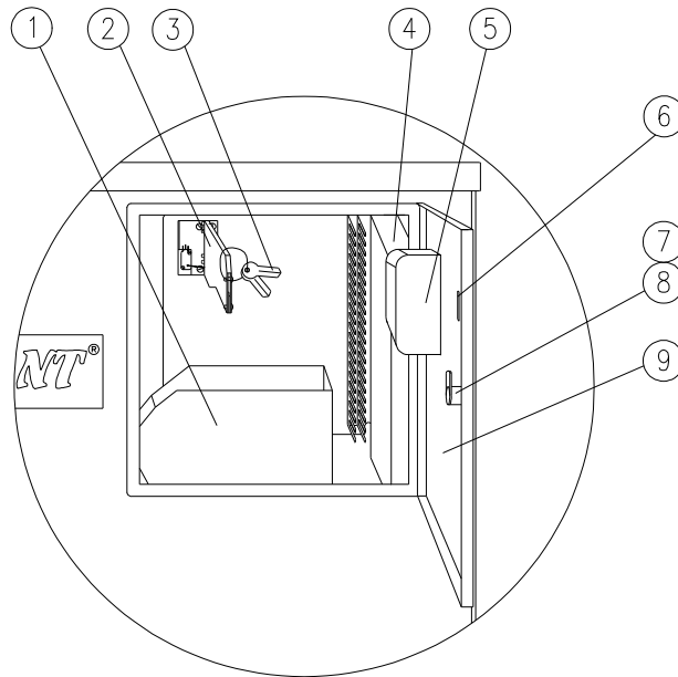
Figur 28: Elskåp
