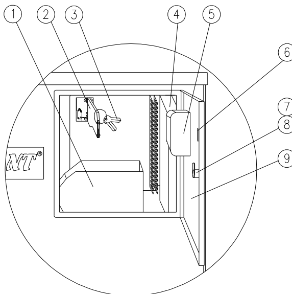
Figure 38: Armoire électrique
