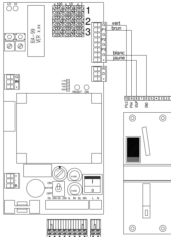
Figure 30: Branchement du contrôle de pièces de monnaie MARS® Cashflow 340.
