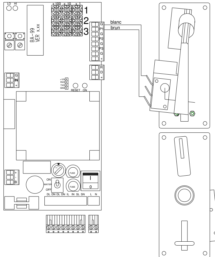
Figure 28: Schéma de branchement, contrôle mécanique des pièces de monnaie, une pièce
