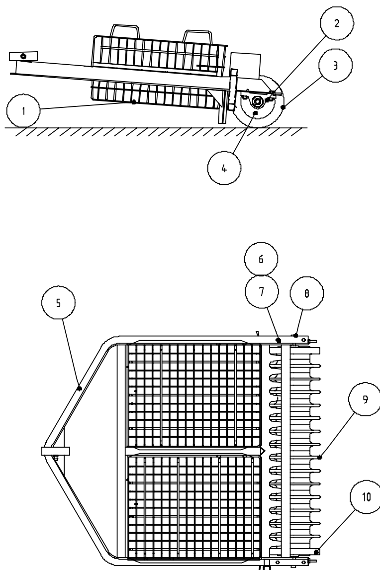
Figur 10: Plocksektion, multiflex
