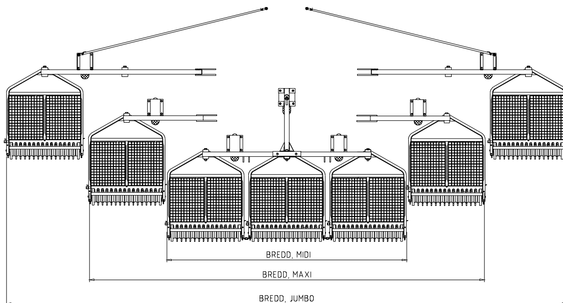
Figur 2: Bollplockarens bredd
